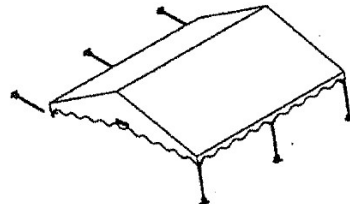
⑥ - Ancrages des pieds et haubannages
