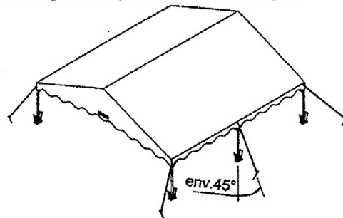
⑥ - Ancrages des pieds et haubannages
